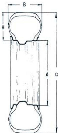
Figuur 11.2 Dwarsdoorsnede en maataanduidingen van landbouwbanden.
