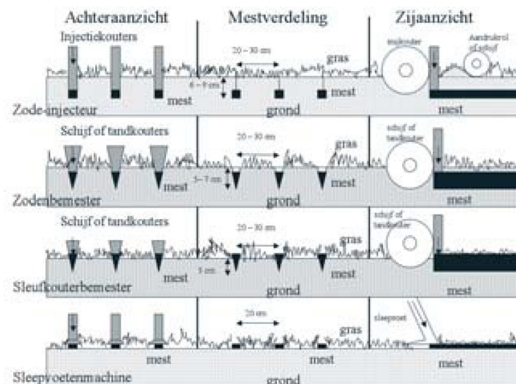
Figuur 11.3 Mestverdeling bij emissiearme mesttoedieningstechnieken op grasland.
