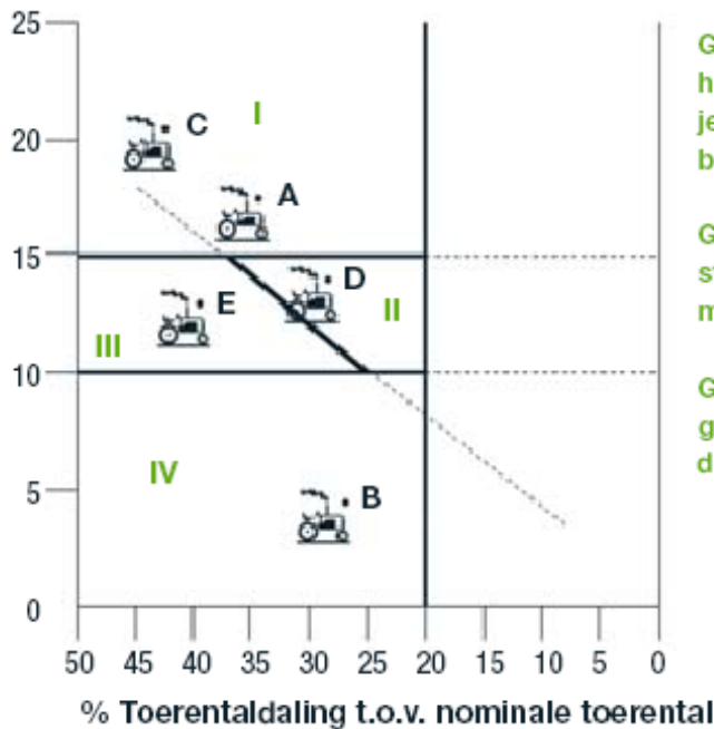
Figuur 11.1 Diagram ter beoordeling of een trekker onder plotseling zware omstandigheden hapert bij toerendaling.
