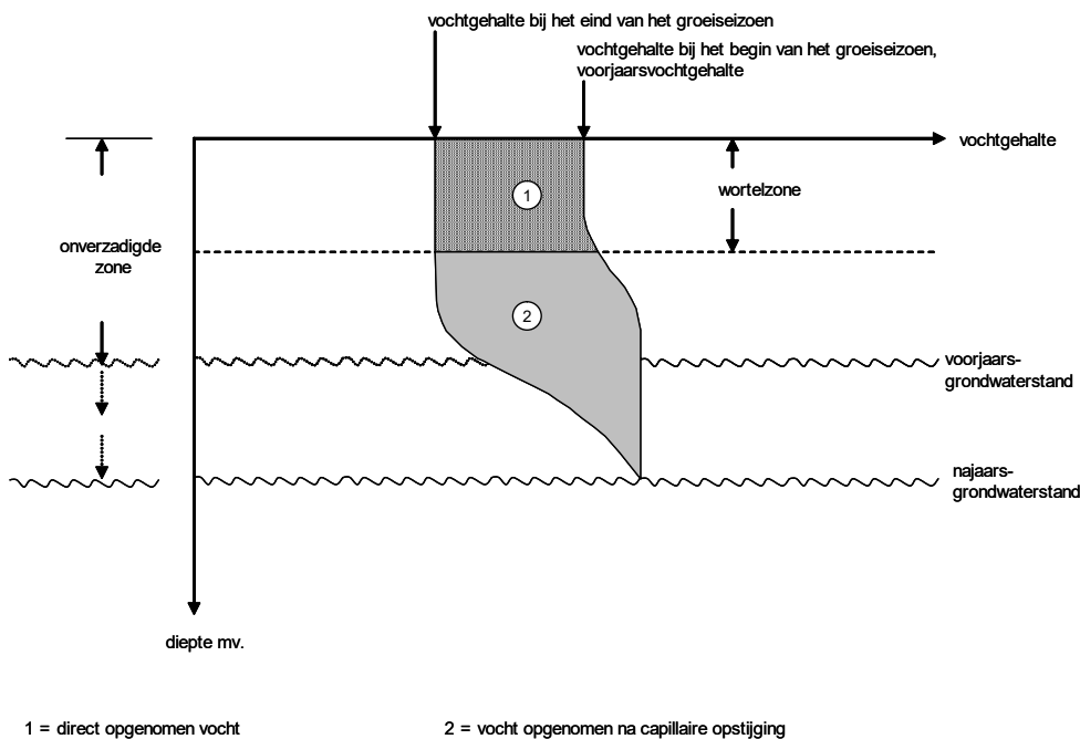
Figuur 1.4 Schematische weergave van de uitdroging van de bodem door vochtname door een gewas tijdens een droog zomerseizoen (Wesseling, 1976).
