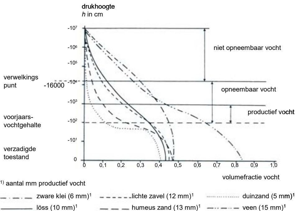
Figuur 1.3 Vochtkarakteristieken van monsters van zes verschillende grondsoorten.
