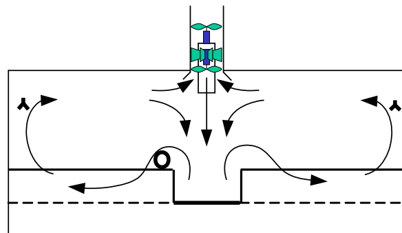
Dwarsdoorsnede combiventilatie
