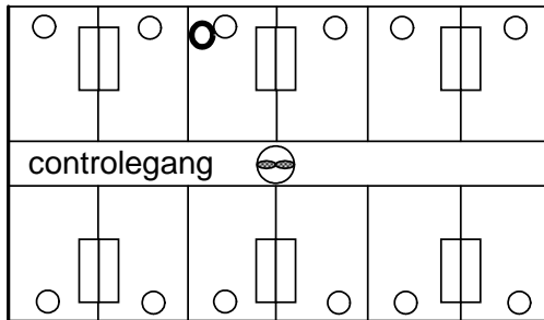
Plattegrond buisventilatie
